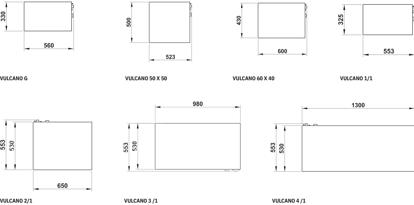
Disegno tecnico - Technical drawing
