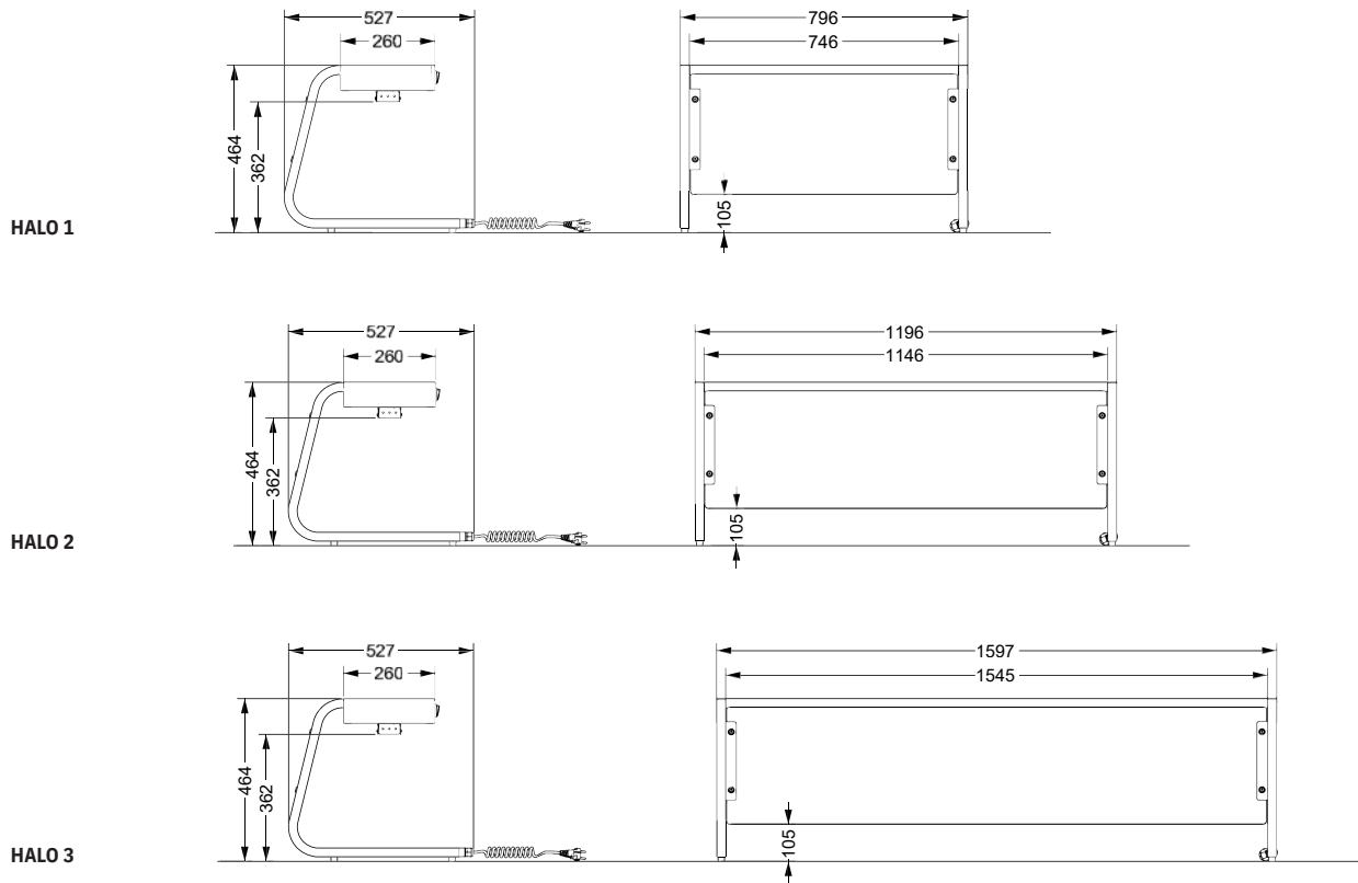
Disegno tecnico - Technical drawing
