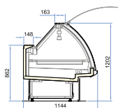
Dream LX P90 TCS
