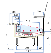
Dream ST P90 / H113 HUR L93-125-188-250-312-375-AE-AI
