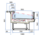
Self ST P90 TN L93-125-188-250-312-375-AE-AI
