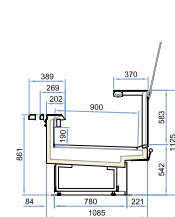
Dream ST P90 / H113 N L93-125-188-250-312-375-AE-AI
