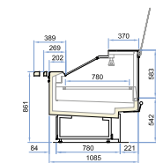
Dream ST P90 / H113 TCS L93-125
