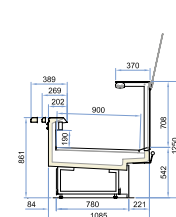
Dream ST P90 / H125 N L93-125-188-250-312-375-AE-AI
