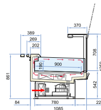
Dream ST P90 / H125 TN L93-125-188-250-312-375-AE-AI
