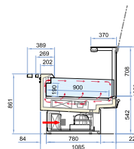
Dream ST P90 / H125 HUR L93-125-188-250-312-375-AE-AI
