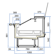
Dream ST P90 / H113 TCB L93-125
