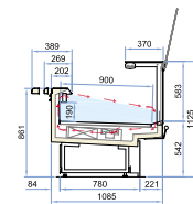
Dream ST P90 / H113 TN L93-125-188-250-312-375-AE-AI
