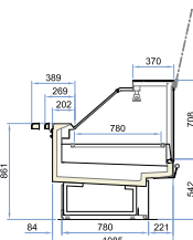
Dream ST P90 / H125 TCS L93-125
