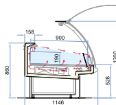
Dream LX P90 HUR
