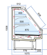
Globe ST H150 L125-188-250-375
