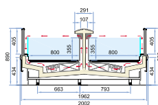
Script L250-375
