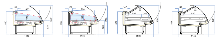
Wing LX P90 TN L93-125-188-250-312-375-AE-AI
